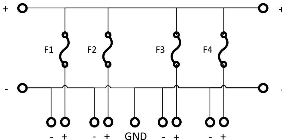
Diagrama de cableado interno del Lynx Distributor
