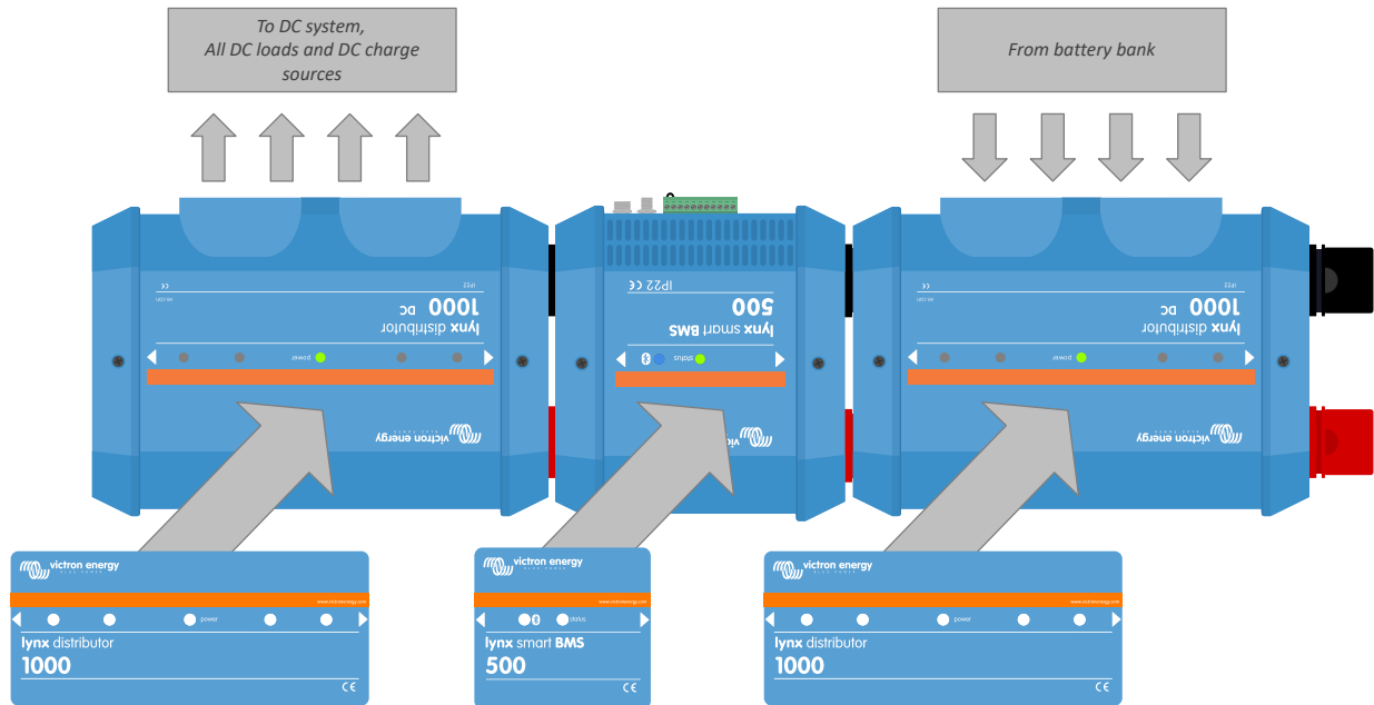
Ejemplo de módulos Lynx montados boca abajo: las baterías se conectan en el lado derecho, todas las cargas y los cargadores se conectan en el lado izquierdo y se colocan las pegatinas correspondientes.
