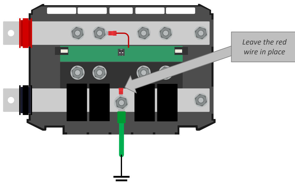
Conexión a tierra Lynx Distributor
