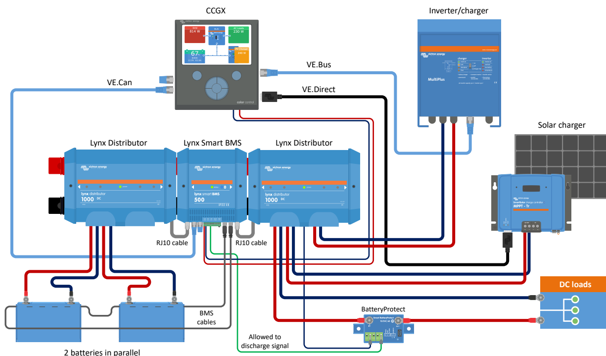
Sistema con baterías de litio, Lynx Smart BMS y dos distribuidores Lynx
